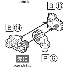
〈ジョイントB〉 Joint B
